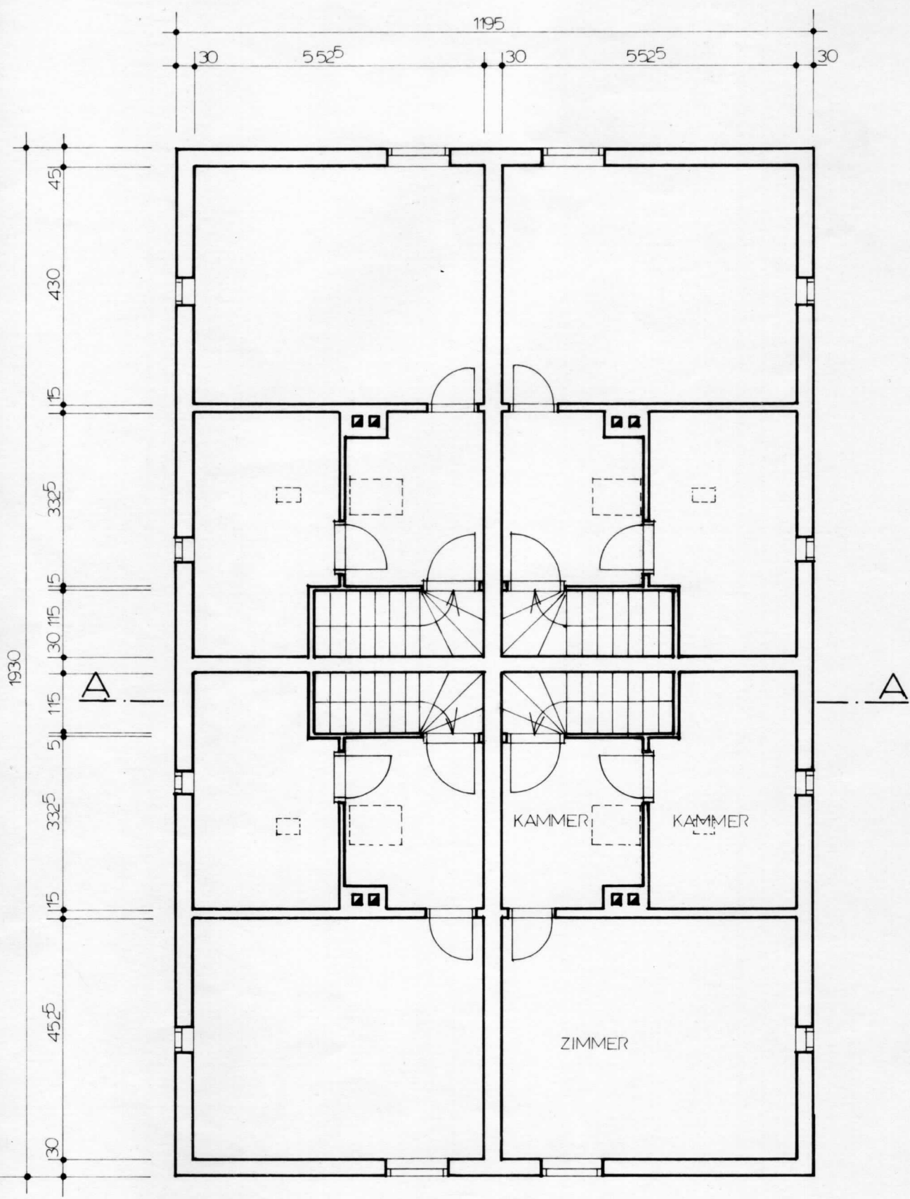
DACHGESCHOSS
