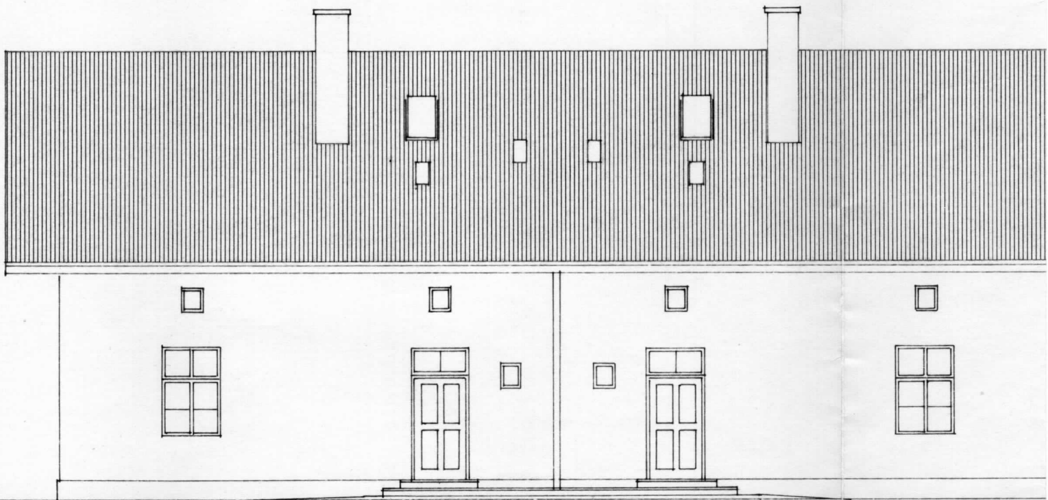
GARTENANSICHT
