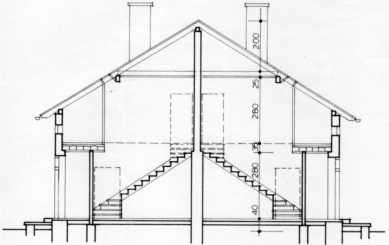
SCHNITT AA
