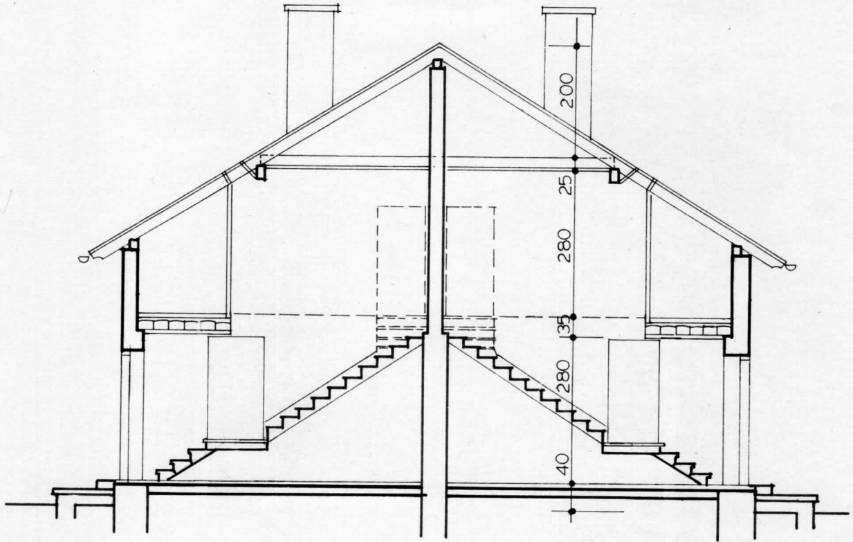
SCHNITT AA
