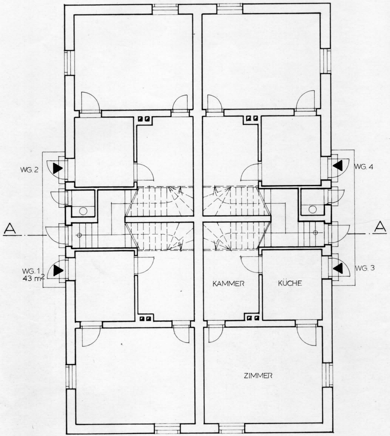
ERDGESCHOSS
