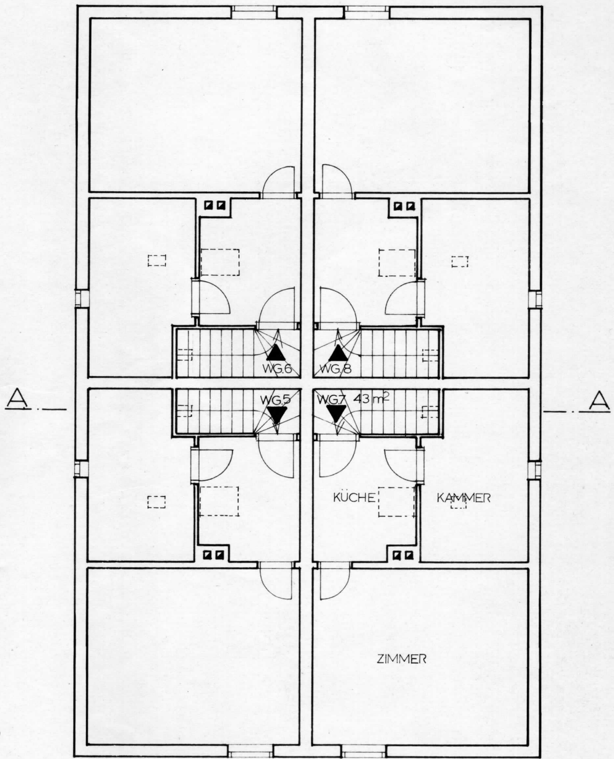
DACHGESCHOSS
